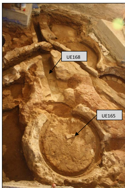
Fotografia 36. Vista general de la premsa UE165 amb la canalització per desaiguar UE168.
